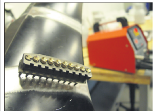
PinPull bliver hæftet let på metallet med en svejsestrøm og kan herefter trække bulen ud med forskellige adaptere.
